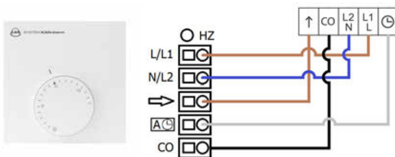
Рис. 63. Схема клемм и подключения термостата отопления/охлаждения Basic+ 230 или 24 В (с возможностью периодического изменения температуры путем подключения таймера)
