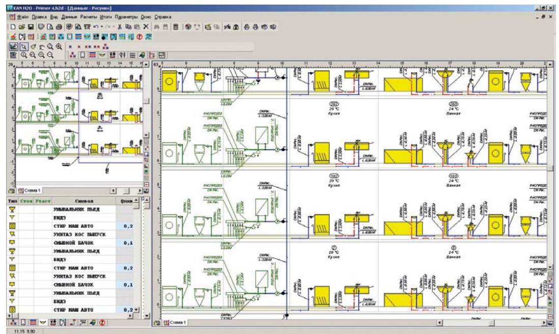
Схема системы водоснабжения в программе KAN H2O
