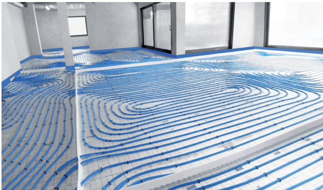
Рис. 24. Напольное отопление, выполненное в системе KAN-therm Tacker
